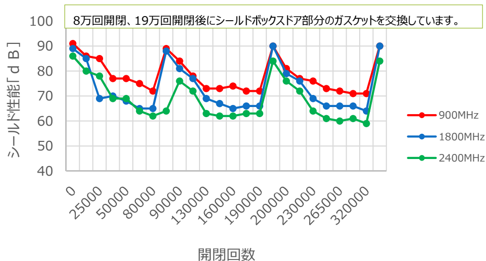
TC-5901C シールドボックス シールド性能 耐久検査
